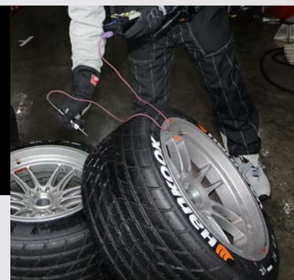
1 물체의 표면 온도를 재는 적외선 온도계. 2 케이블 탐침식 온도계. 내열 케이블을 사용하면 오븐 속 온도를 잴 수 있다. 3 오븐 속에 넣는 아날로그 온도계. 4 국이나 수프 같은 액체라면 어디든 사용할 수 있는 튀김용 온도계. 5 무선 알람(소리/진동) 장치가 딸린 탐침식 디지털 온도계. 6 냉장/냉동고용 온도계. 센서는 안에 넣고 온도계는 냉장고 표면에 붙일 수 있다. 7, 8, 9, 10 가장 기본적인 탐침식 온도계. 탐침 보호 커버가 제공된다. 11 K-타입 센서 플러그를 교체하면 다양도로 사용할 수 있는 정밀 온도계(주방에서 사용할 수 있는 탐침식 센서도 있다). 한국타이어 모터스포츠 지원 팀이 서킷 피트에서 타이어 표면 온도를 잴 때도 이렇게 생긴 온도계를 사용한다.
